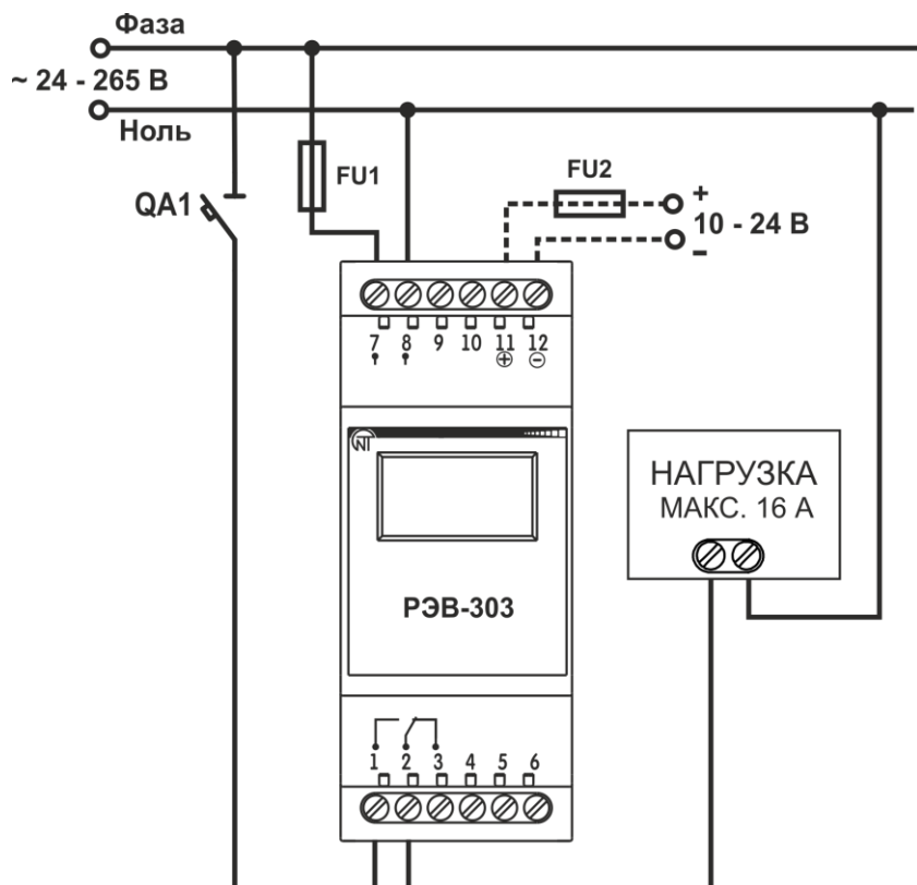
QA1 - Автоматический выключатель (макс. 16 А); FU1, FU2 - Плавкий предохранитель (макс. 1 А).
