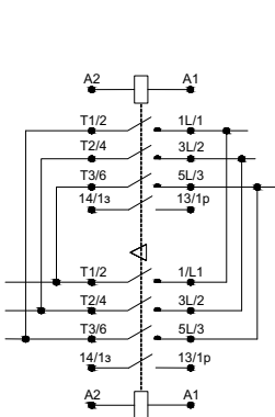
Рисунок 1 – Электрические принципиальные схемы для контакторов КМИ-10930, КМИ-11230, КМИ-11830, КМИ-22530, КМИ-23230 / Figure 1 – Electrical circuit diagrams for KMI-10930, KMI-11230, KMI-11830, KMI-22530, KMI-23230 contactors
