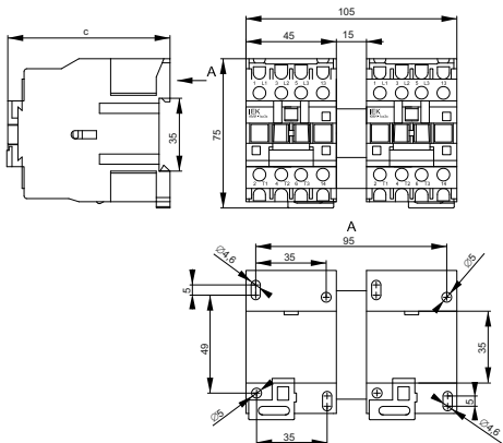
Рисунок 3 – Габаритные и установочные размеры КМИ-10930, КМИ-11230, КМИ-11830 / Figure 3 – Overall and installation dimensions of KMI-10930, KMI-11230, KMI-11830
