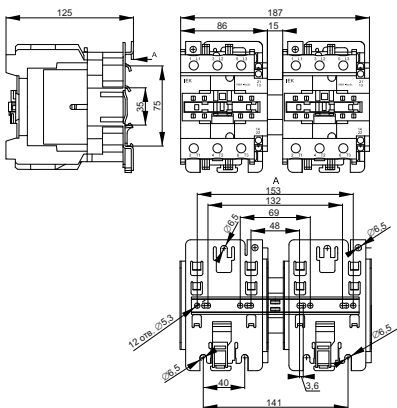
Рисунок 6 – Габаритные и установочные размеры КМИ-48032, КМИ-49532 / Figure 6 – Overall and installation dimensions of KMI-48032, KMI-49532
