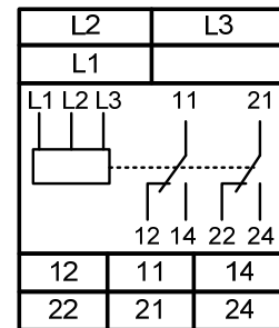
Схема подключения
