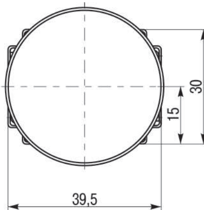
Рисунок 1 - Габаритные и присоединительные размеры кнопок
