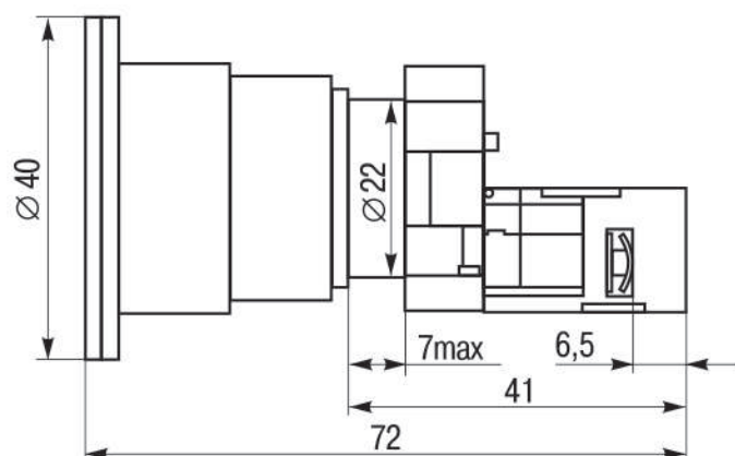
Рисунок 1 - Габаритные и присоединительные размеры кнопок
