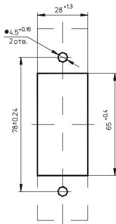
Рисунок Б.3 - Сверление отверстий под винты крепления выключателя
