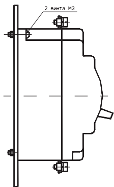
Рисунок Б.2 Крепление выключателя
