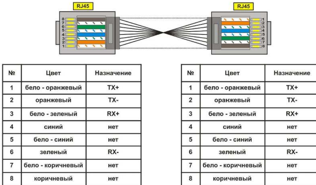
Рисунок 5.3 – Нумерация выводов кабеля соединения с сетью Ethernet
