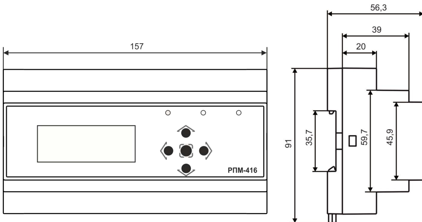
Рисунок 1.1 – Внешний вид и габаритные размеры регистратора
